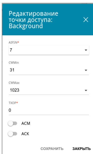
Рисунок 89. Окно для изменения параметров функции WMM.
