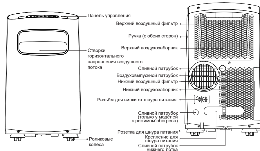
Вид спереди
