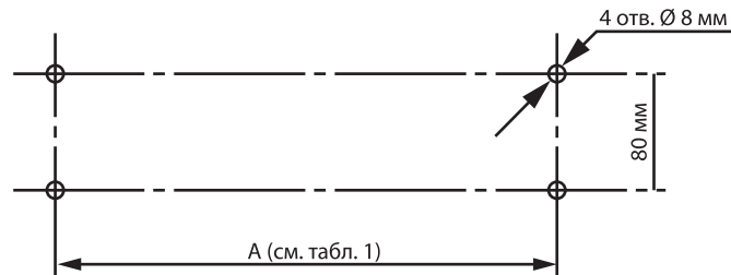
Рис. 1 Схема разметки отверстий
