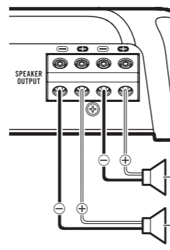
Выход громкоговорителя
