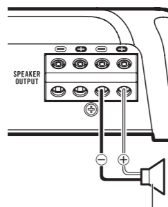
Выход громкоговорителя
